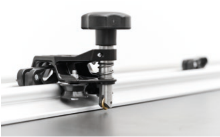
Si raccomanda di usare strumenti professionali: una guida di taglio provvista di ventose incorporate e di incisore con rotellina in titanio.
